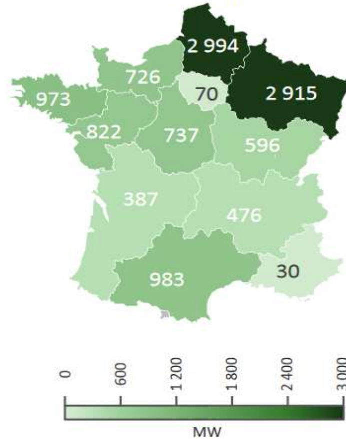
Répartition des capacités de production éolienne
