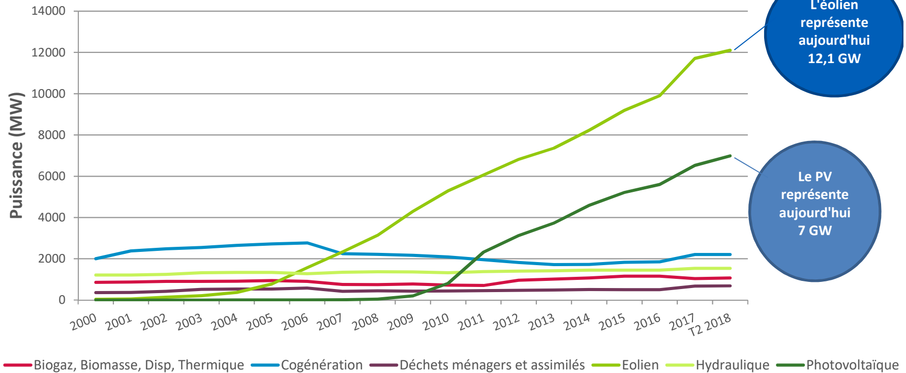
Installations raccordées au réseau public de distribution géré par Enedis
