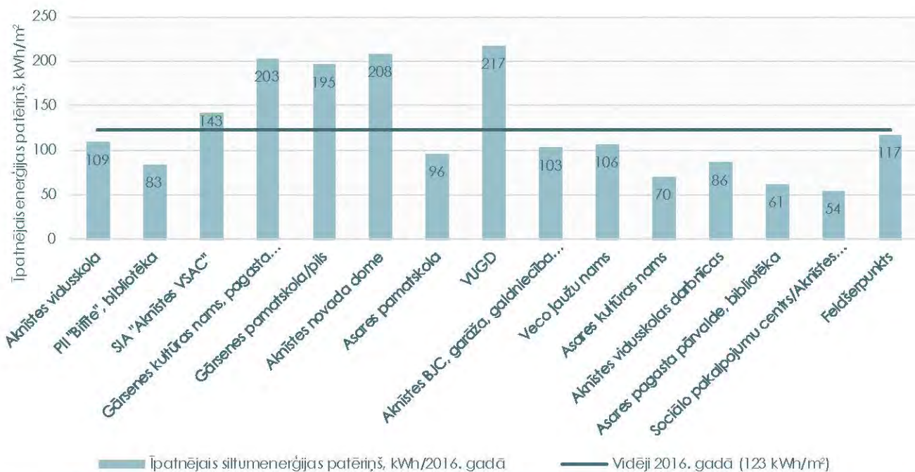
2.19. ATTĒLS: Īpatnējais siltumenerģijas patēriņš (kWh/m²) pašvaldības ēkās Aknīstes novadā 2016. gadā. (Pilnie ēku nosaukumi: SIA Aknīstes veselības un sociālās aprūpes centrs, Gārsenes kultūras nams un pagasta pārvalde, Aknīstes B.J.C. garāža, galdniecība (Aknīstes kultūras centrs), Sociālo pakalpojumu centrs/Aknīstes senioru centrs)
