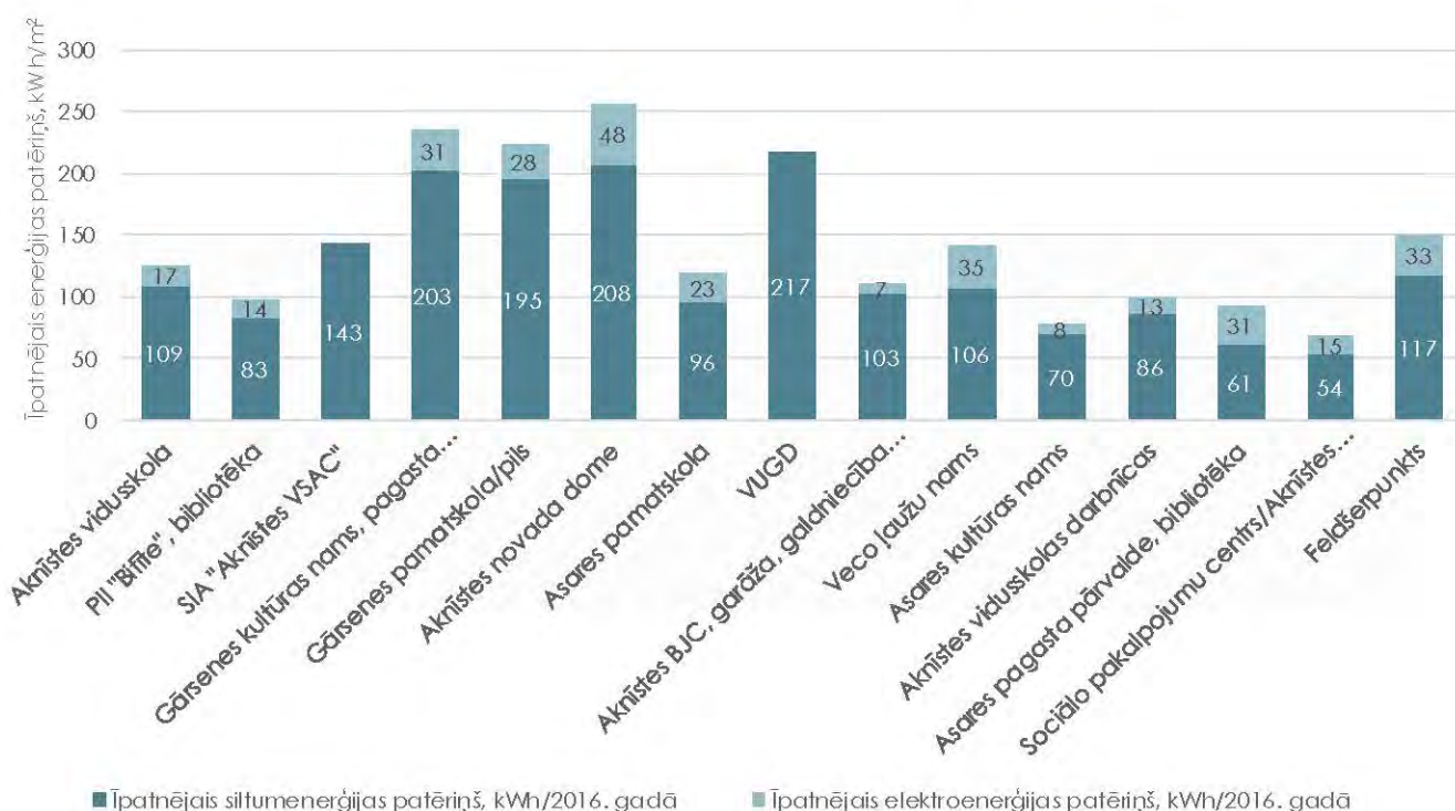
5.1. Attēls: Īpatnējais siltumenerģijas un elektroenerģijas patēriņš pašvaldības ēkās Aknīstes novadā 2016. gadā
