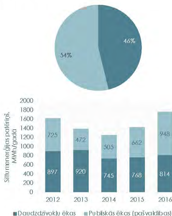
2.15. ATTĒLS: CSS siltumenerģijas patēriņa sadalījums atkarībā no patērētāja grupas pa gadiem un 2016.gadā.
