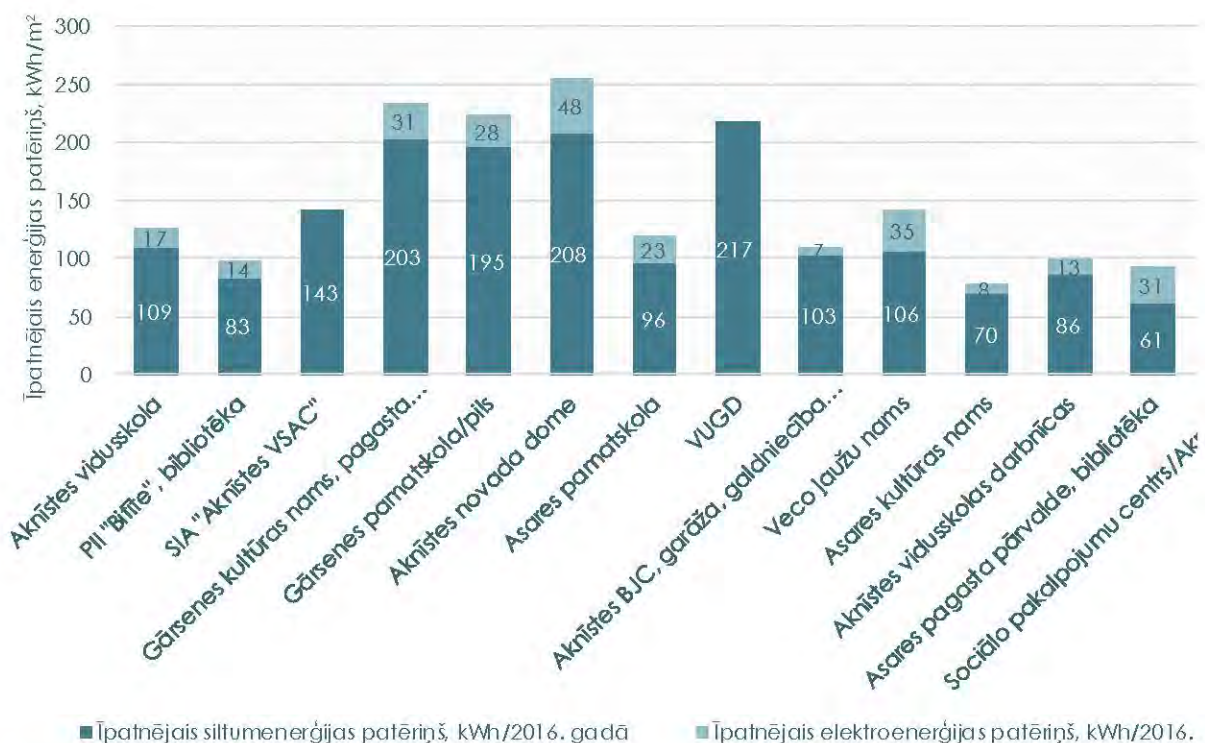
2.18. ATTĒLS: Siltumenerģijas un elektroenerģijas patēriņš pašvaldības ēkās Aknīstes novadā 2016. gadā. (Pilnie ēku nosaukumi: SIA Aknīstes veselības un sociālās aprūpes centrs, Gārsenes kultūras nams un pagasta pārvalde, Aknīstes BJC, garāža, galāniecība (Aknīstes kultūras centrs), Sociālo pakalpojumu centrs/Aknīstes senioru centrs)
