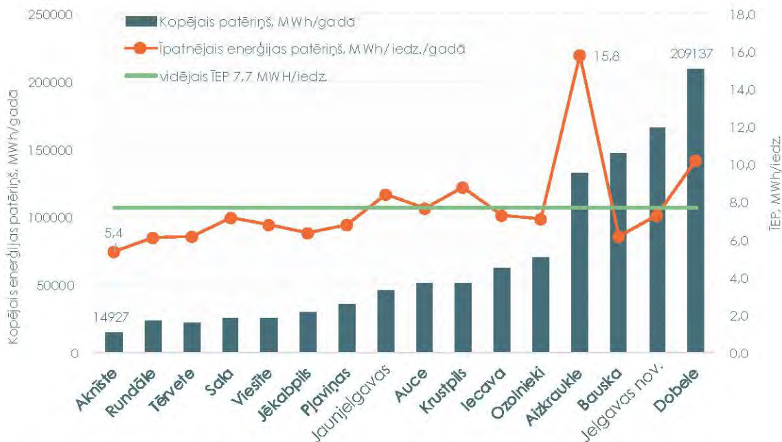
2.30. ATTĒLS: Kopējais īpatnējais enerģijas patēriņš Zemgales plānošanas reģiona novados 2016. gadā, MWh/I iedzīvotāju gadā
