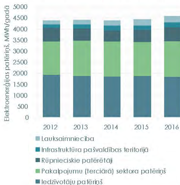
2.22. ATTĒLS: Elektroenerģijas patēriņš Aknīstes novadā
