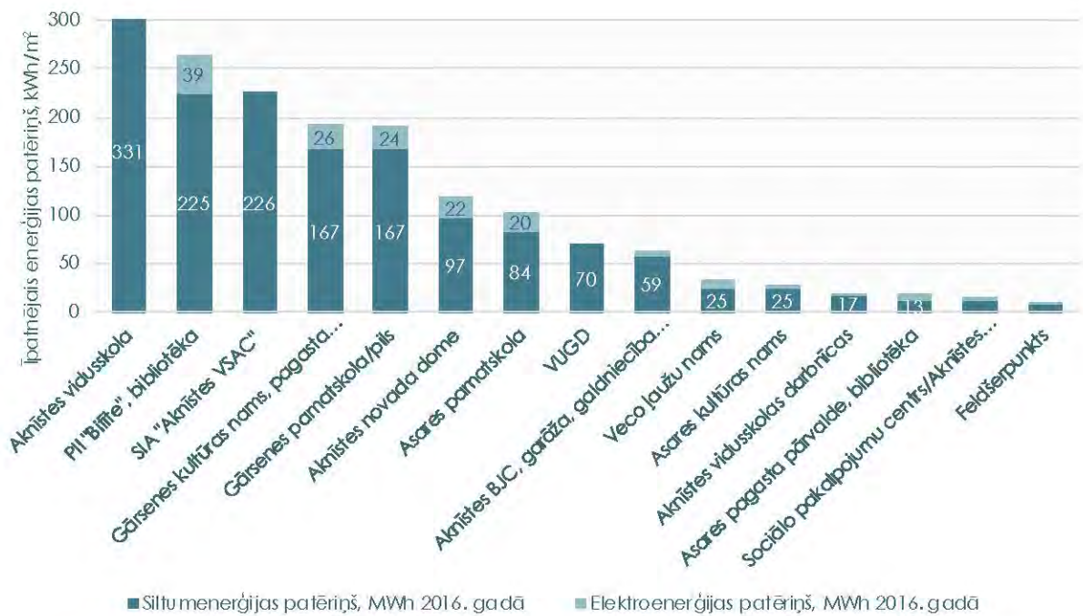
2.23. ATTĒLS: Siltumenerģijas un elektroenerģijas patēriņš pašvaldības ēkās Aknīstes novadā 2016. gadā. (Pilie ēku nosaukumi: SIA Aknīstes veselības un sociālās aprūpes centrs, Gārsenes kultūras nams un pagasta pārvalde, Aknīstes BJC, garāža, galdniecība (Aknīstes kultūras centrs), Sociālo pakalpojumu centrs/Aknīstes senioru centrs)
