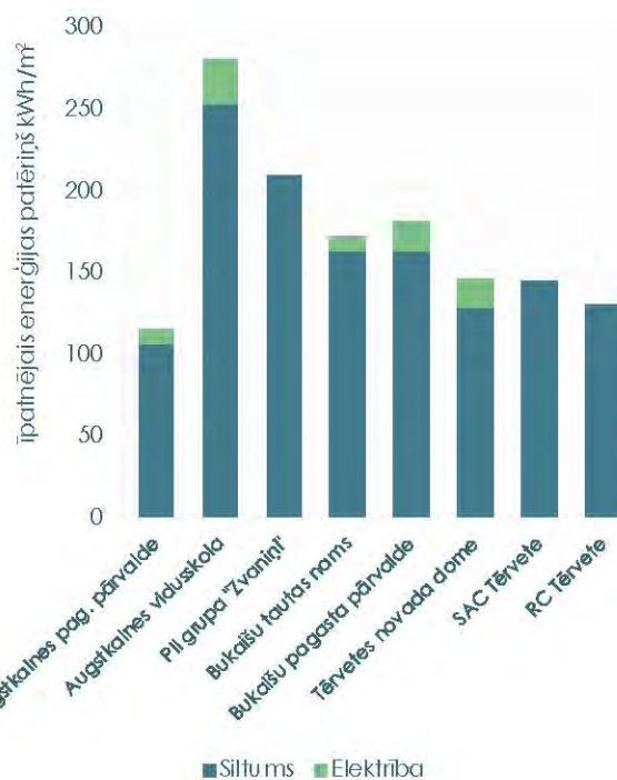
2.11. ATTĒLS: Tērvetes novada pašvaldības ēku īpatnējais enerģijas patēriņš 2016. gadā
