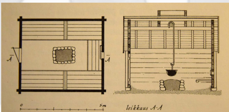
Pohjakuva ja pitkittäisleikkaus Sumisaaren kodasta Kenttäsaaresta (Anttila 1965)
