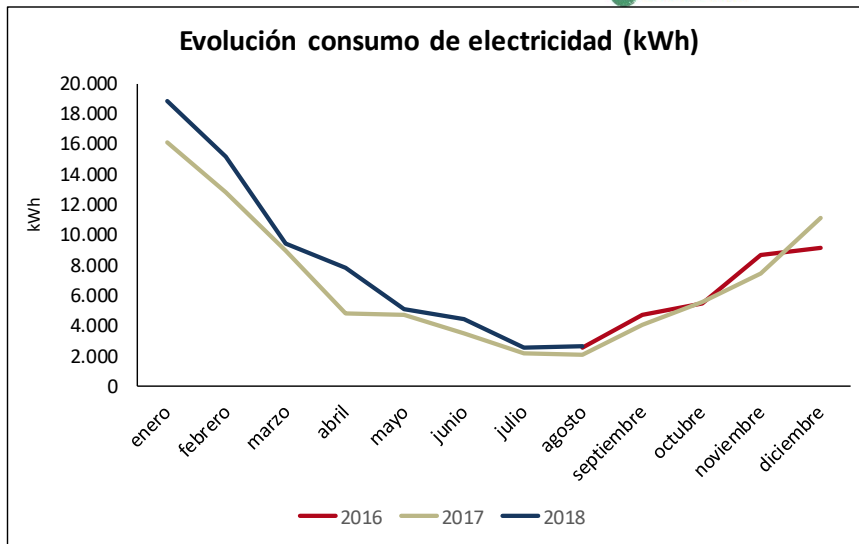
Gráfica 8. Evolución del consumo eléctrico (2016-2018)
