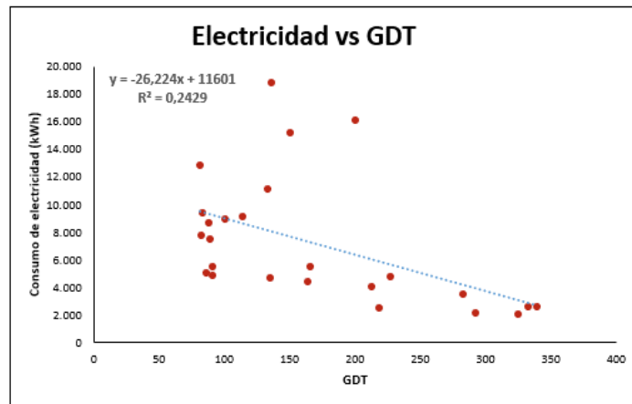
Gráfica 9. Regresiones lineales para establecer la línea base de electricidad
