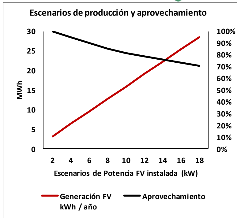
Gráfica 11. Escenarios de generación FV y aprovechamiento
