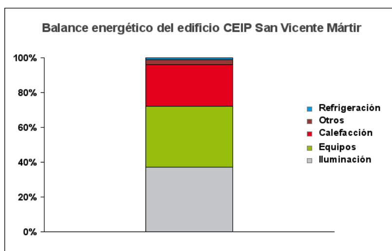
Gráfica 5. Balance energético por usos
