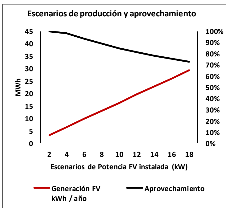
Gráfica 9. Escenarios de generación FV y aprovechamiento
