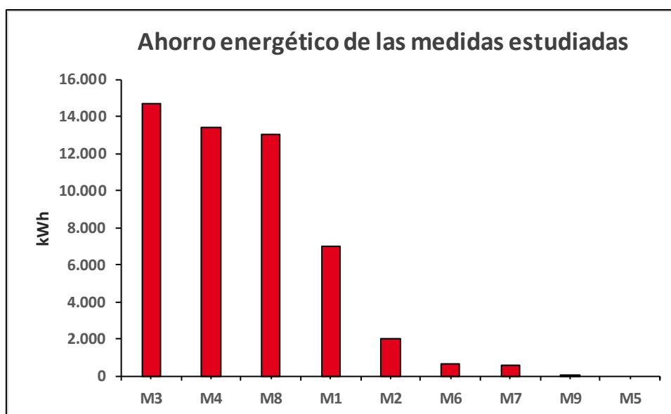
Gráfica 11. Ahorro energético anual de las medidas de ahorro estudiadas
