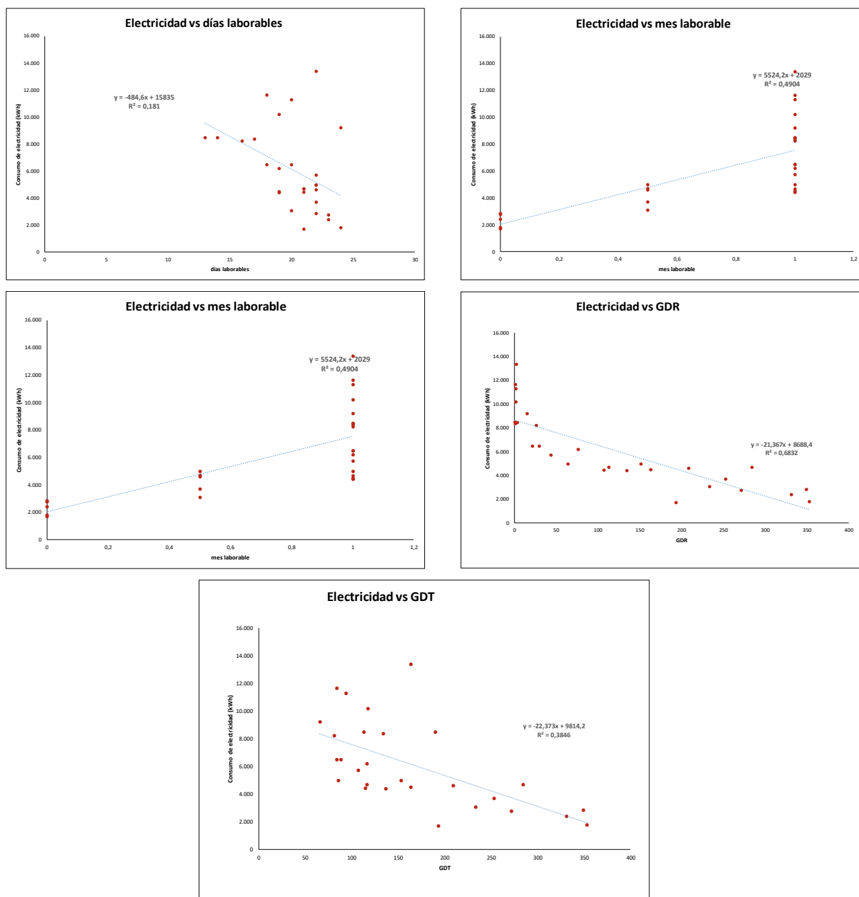
Gráfica 7. Regresiones lineales para establecer la línea base de electricidad
