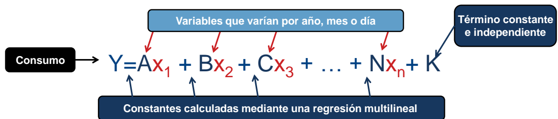
Ilustración 9. Función multivariable
