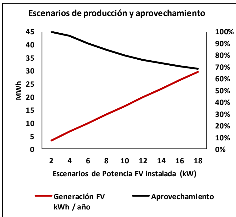
Gráfica 10. Escenarios de generación FV y aprovechamiento
