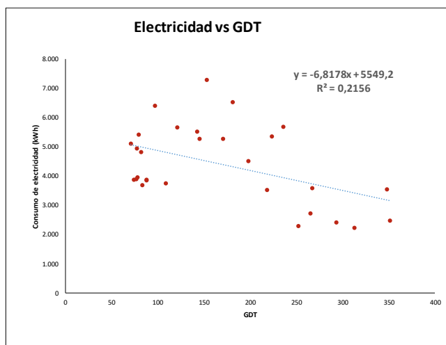
Gráfica 8. Regresiones lineales para establecer la línea base de electricidad
