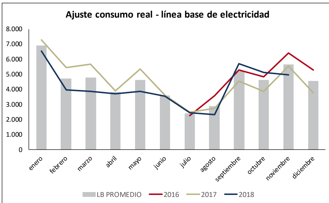
Gráfica 9. Ajuste de la línea base y el consumo real
