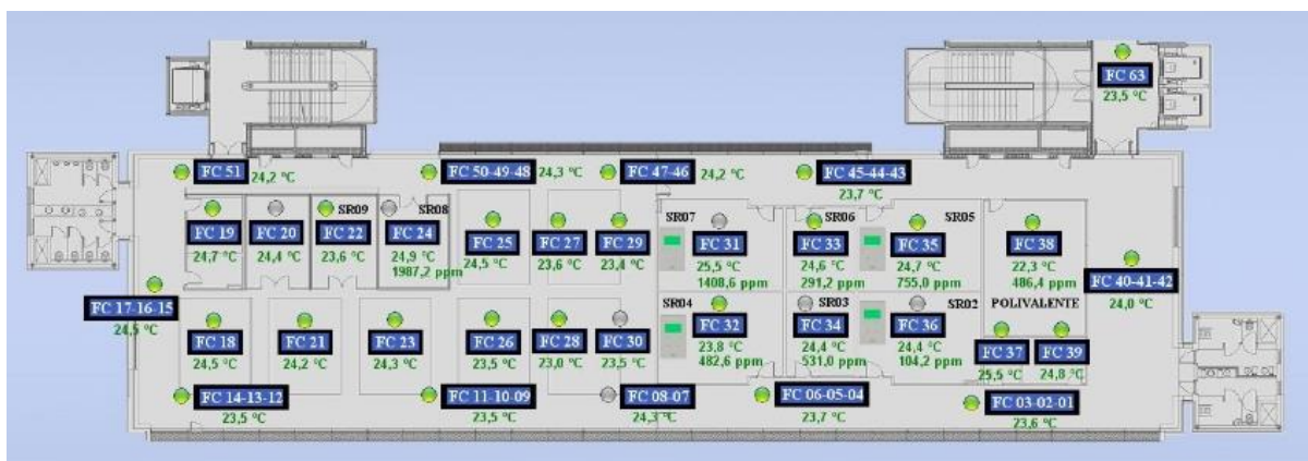
Ilustración 17. Ejemplo de un Sistema de Control Centralizado para climatización
