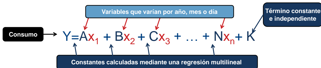
Ilustración 9. Función multivariable
