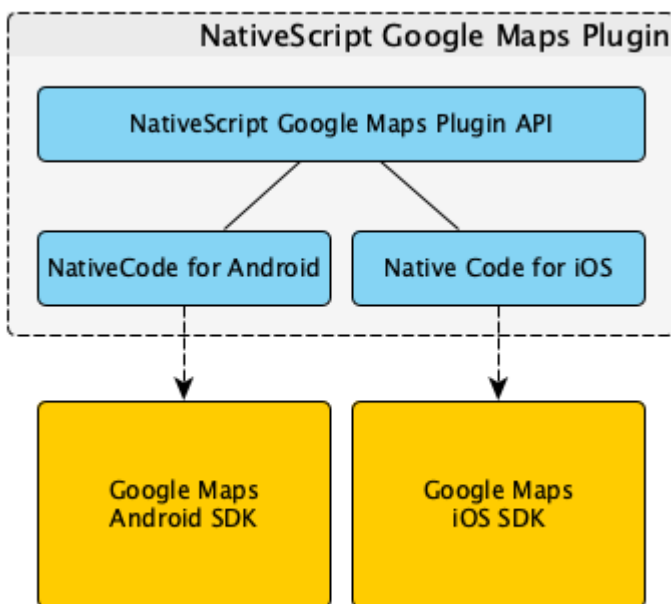
Fig. 13 - Architettura di un plugin NativeScript
