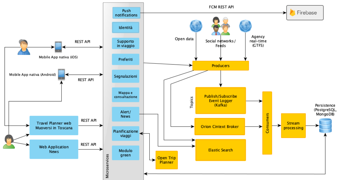
Fig. 1 - Architettura della piattaforma Muoversi In Toscana
