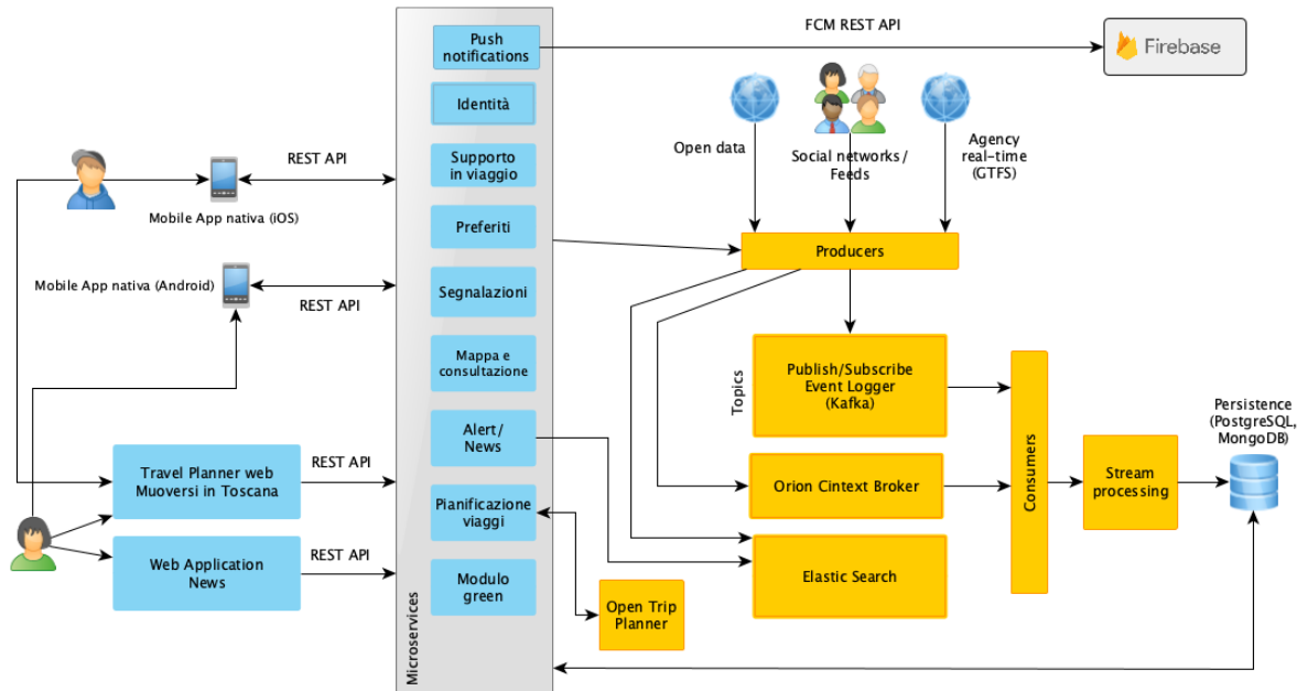
Fig. 7 - Architettura della piattaforma Muoversi In Toscana
