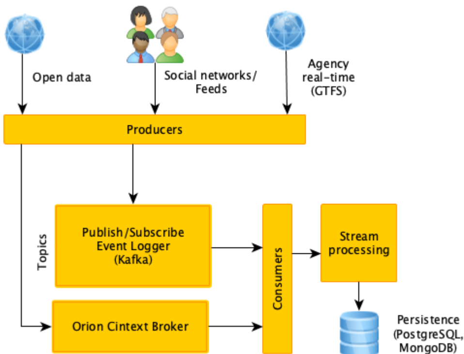
Fig. 10 - Stream processing dei dati di terze parti
