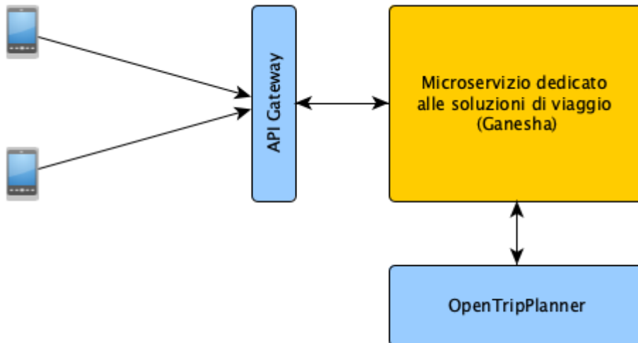
Fig. 2 - Servizio dedicato alla pianificazione viaggi
