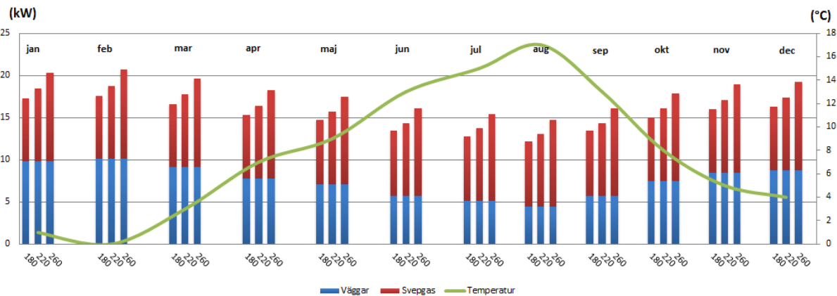
Figur 14: För varje månad presenteras värmeförbrukningen för svepgasflödena 180, 220 och 260 m 3 /h i kW. Utomhustemperaturerna ges av kurvan i °C och baserades på SMHI:s data för Töreboda år 2015.
