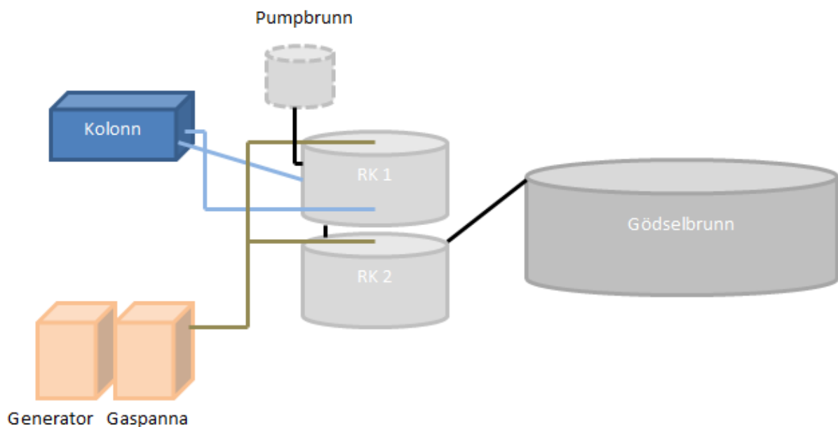
Figur 4: Biogasanläggningen vid Sötåsen. Pumpbrunnen ligger under marken
