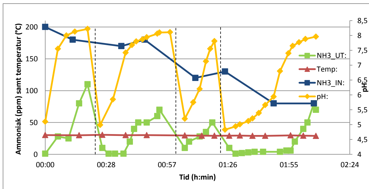
Figur 13: Grafen visar hur NH 3 in i och ut ur skrubbern samt pH och temperatur varierade med tiden. När en streckad linje korsar två mätpunkter betyder det att pH i tvättvätskan har justerats ned under tiden mellan de två mätpunkterna.
