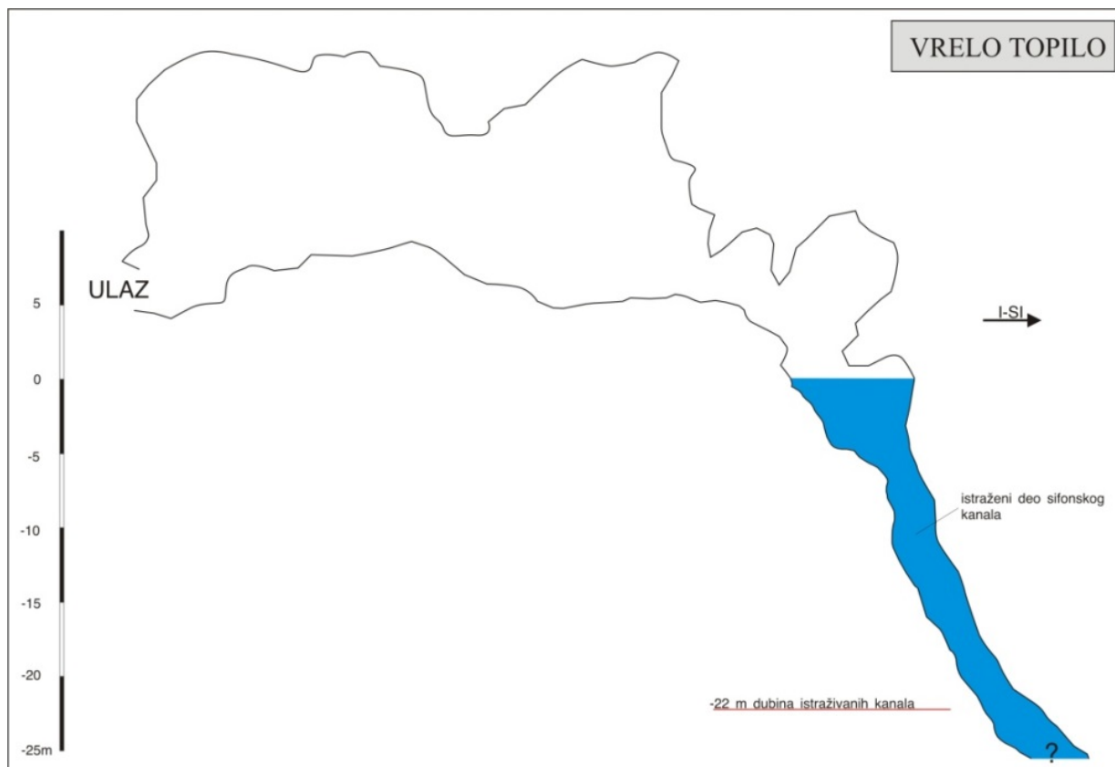
Слика 6: Врело Пештер (Топило) – профил (Милановић С., 2012)
