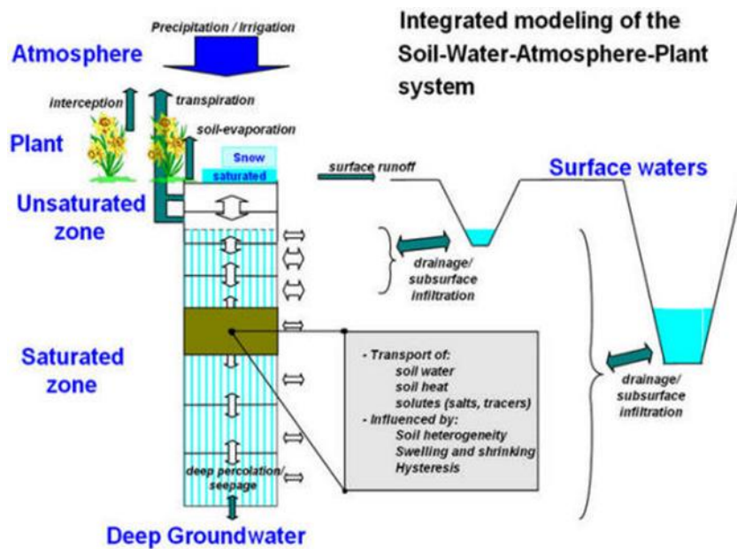
Figuur 23: Schematische weergave van het met SWAP gemodelleerde domein (Kroes et al., 2017)
