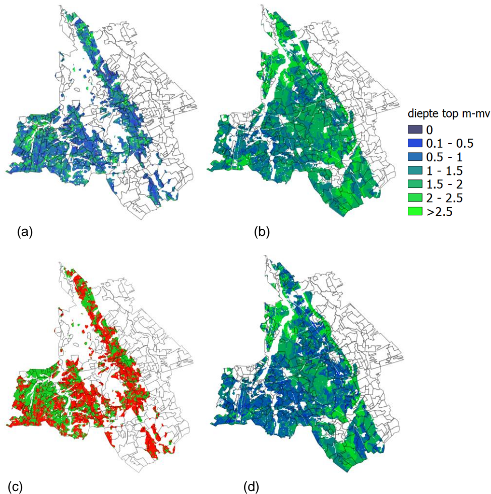
Figuur 24: a. diepte van de bovenkant van de keileemlaag in de MIPWA keileemkaart. b. Diepte van de bovenkant van de keileemlaag in de 74 verdiepte bodemprofielen. c. Locaties waar de keileemkaart van MIPWA een keileemdikte geeft die meer dan 20 cm hoger ligt dan het geval is voor de 74 verdiepte bodemprofielen (in rood). Voor deze gebieden zijn extra profielen aangemaakt waarbij de keileemdikte is aangepast. d. Diepte van de bovenkant van de keileemlaag voor de 74 profielen met 37 aangepaste profielen op basis van de keileemkaart. Dit resulteert in 111 bodemprofielen.
