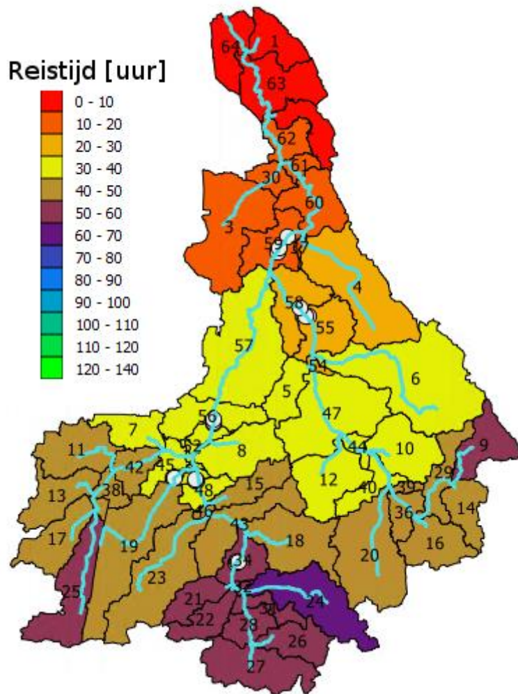
Figuur 19. Cumulatieve reistijd bij hoge afvoer ( 7 \text{ m}^3 \text{ s}^{-1} ) van de piekconcentratie van een conservatieve opgeloste stof in de waterlopen van de Drentsche Aa naar het station De Punt in het noorden van het gebied. De reistijd voor elk substroomgebied is inclusief de reistijd binnen het substroomgebied zelf.
