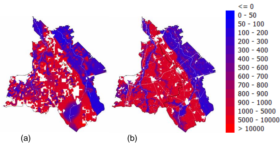
Figuur 27: Drainage weerstand (in dagen) van het afwateringssysteem: a. Alterra kaart, b. mediaan per bodemprofiel. De hoge waarde van 10,000 heeft geen gevolgen voor de berekeningen in SWAP.
