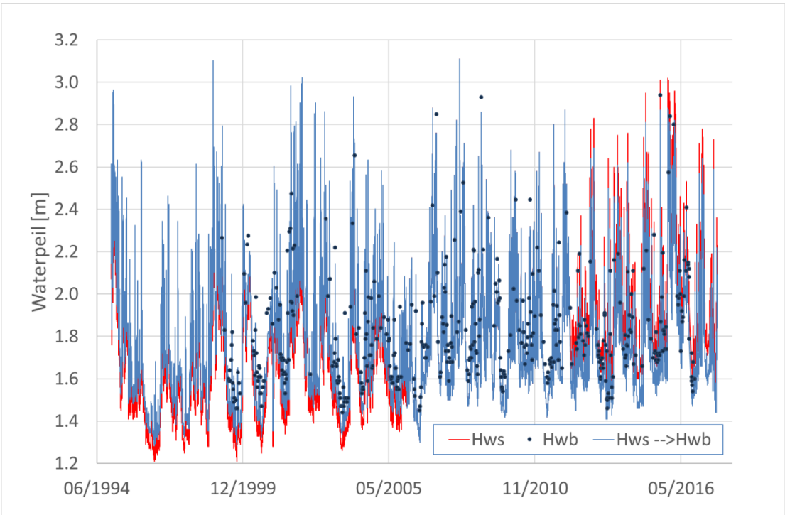
Figuur 2. Originele waterstandreeksen zoals geregistreerd door de drukopnemer van het Waterschap Hunze en Aa's ( H_{ws} ) en de gecorrigeerde reeks ( H_{ws} \rightarrow H_{wb} ) die overeenkomt met de peilschaalwaarden geregistreerd door het Waterbedrijf Groningen ( H_{wb} ). Op alle reeksen moet een correctie naar NAP hoogte gedaan worden van -0,11 m.
