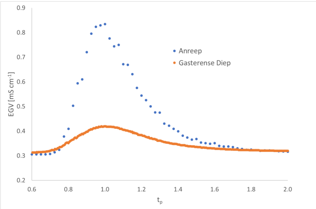
Figuur 20. Dispersie van de instantane injectie van NaCl in de waterloop, zoals gemeten via het elektrisch geleidingsvermogen (EGV). De tijd-as is genormaliseerd door te delen door de tijd van aankomst van de piek ( t_p ).
