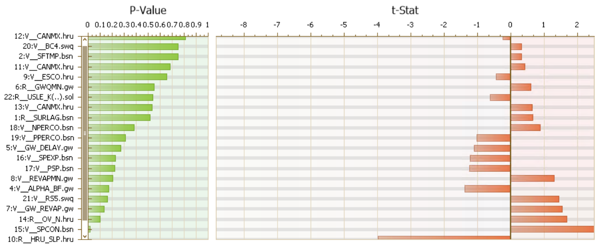
Figuur 64. Statistische significantie van de parameters in een kalibratiestap met SWAT-CUP voor de Hunze.
