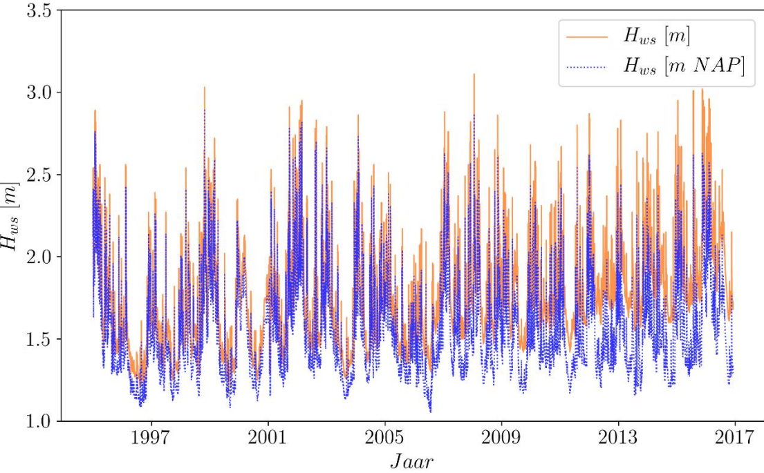
Figuur 3. Originele H_{ws} waterpeilreeksen zoals geregistreerd door het Waterschap Hunze en Aa's, en de gecorrigeerde reeks waarbij de correcties voor verschillen tussen metingen van H_{wb} en H_{ws} , en de correctie ( -0,11 m) voor de meest recente NAP hoogtegegevens van de peilschaal zijn toegepast.
