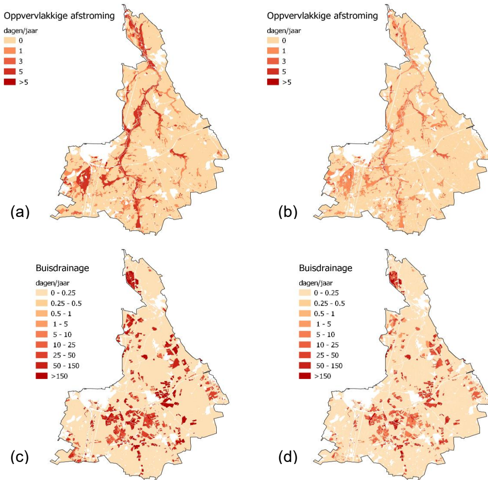
Figuur 31: Het gemiddeld aantal dagen met oppervlakkige afstroming per jaar berekend voor kale bodem (a) en natuur gras (b) in de periode 2003–2008. Hetzelfde voor buisdrainage, voor kale bodem (c) en natuur gras (d).
