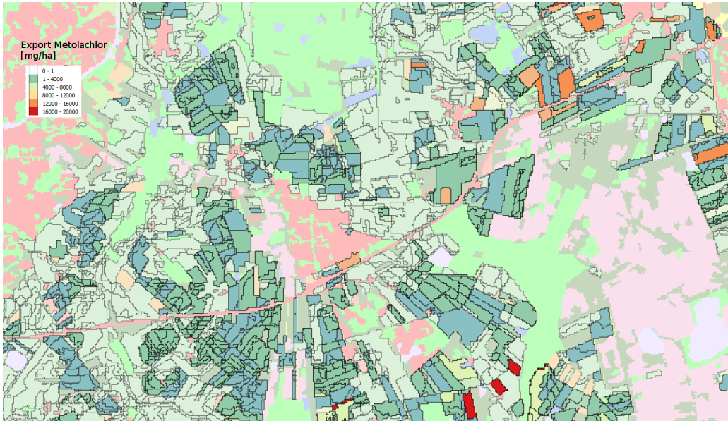
Figuur 74. Detailkaart van de jaarlijkse gemiddelde export van metolachlor uit percelen in de Drentsche Aa (2013-2015).
