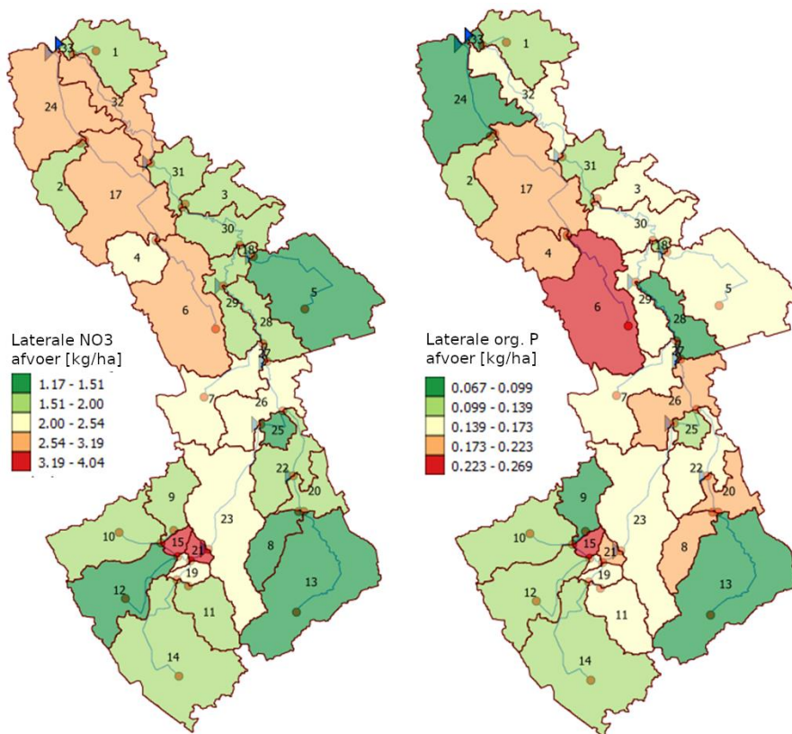
Figuur 79. Laterale afvoer van NO 3 -N en organisch P, zoals gemodelleerd met SWAT voor het stroomgebied van de Hunze (2013-2015).
