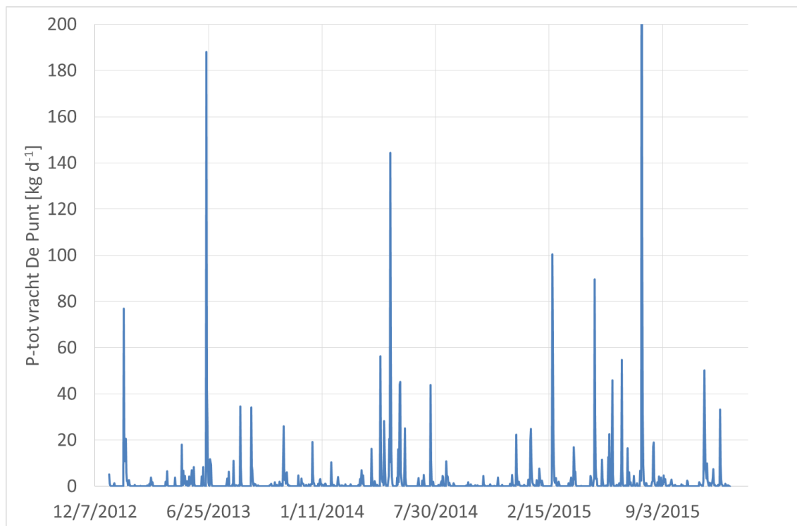
Figuur 69. Vrachten van P-tot bij De Punt voor de jaren 2013-2015. N.B. de y-as is afgekort, waardoor de maximale vracht van 388 kg d -1 in maart 2015 niet is weergegeven.
