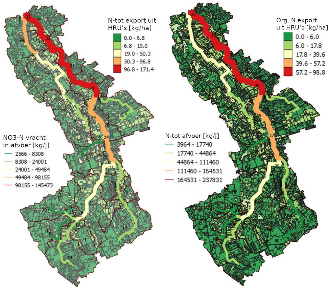
Figuur 80. NO 3 -N en N-tot vrachten in de waterloopsegmenten van de substroomgebieden in het stroomgebied van de Hunze, en N-tot en organisch N export uit de HRU's (2013-2015).
