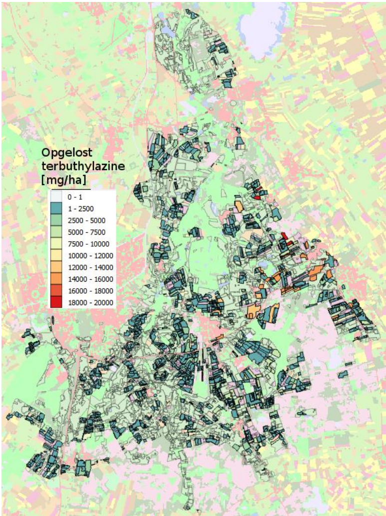
Figuur 73. Jaarlijkse gemiddelde export van terbuthylazine uit HRU's (2013-2015).
