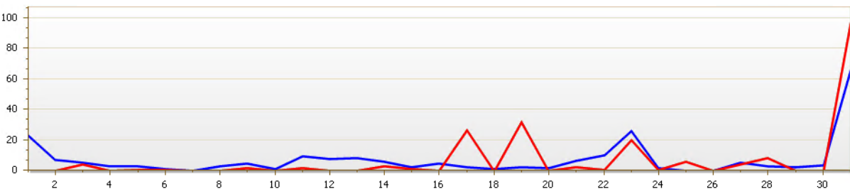
Figuur 62. Kalibratie van P-tot vrachten bij meetpunt Voorste Diep (2013-2015).
