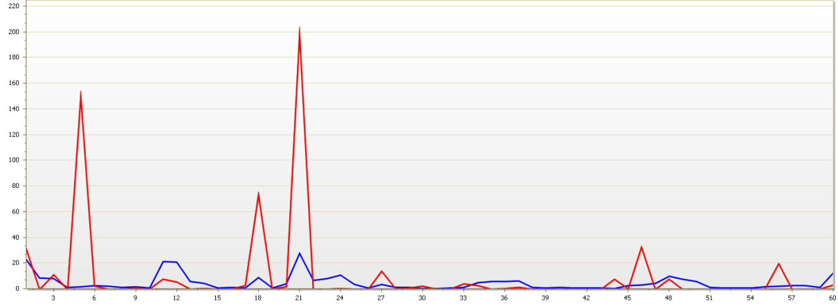
Figuur 53. Kalibratie van de vrachten van mineraal P [ kg d^{-1} ] voor station De Punt ( n=60 ).
