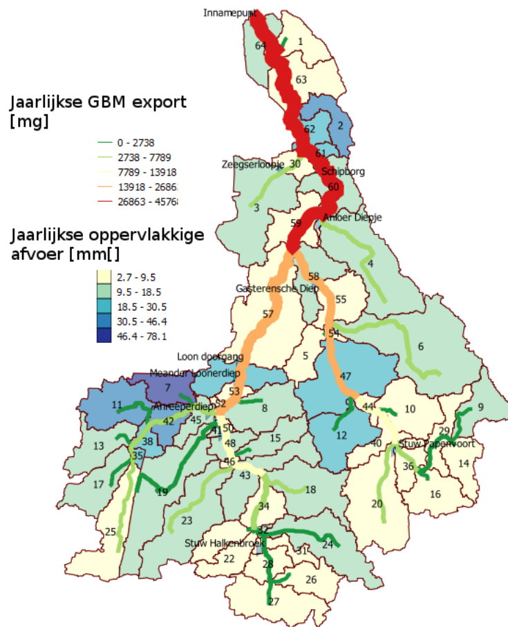
Figuur 72. Jaarlijkse oppervlakkige afvoer vanuit substroomgebieden, en de vrachten van terbuthylazine in de waterlopen van de Drentsche Aa (2013-2015).
