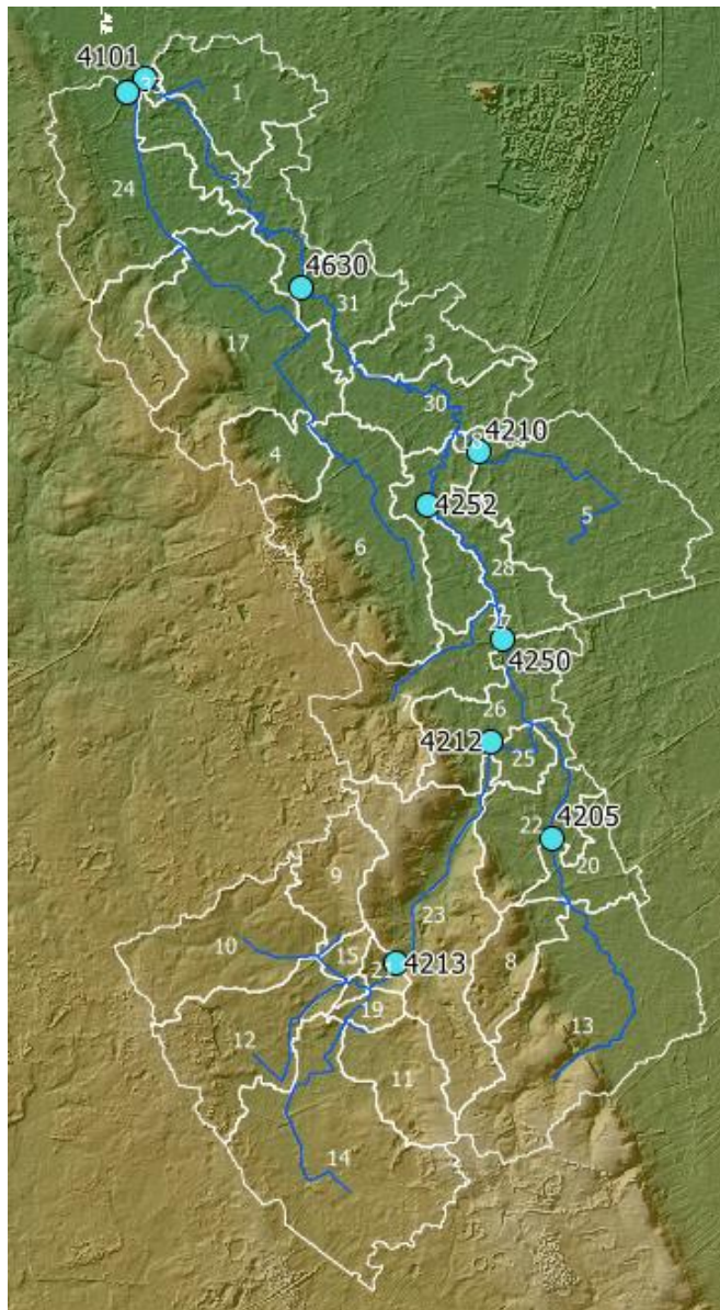
Figuur 42. Indeling van het stroomgebied van de Hunze in sub-stroomgebieden op basis van stroomgebiedsbegrenzing Waterschap Hunze en Aa's, het AHN, hoofdwatervangsten en meetpunten met gebruik van de terreinanalyse routines uit MWSWAT. Meetpunt 4206 ligt ten zuidwesten van punt 4101.
