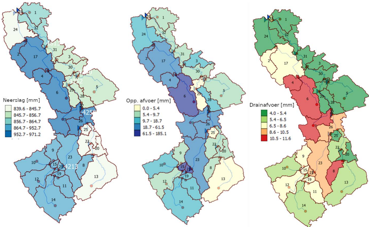
Figuur 76. Ruimtelijke verdeling van de gemiddelde jaarlijkse neerslag, op basis van de invoergegevens van de neerslagmeetstations van het KNMI in het gebied, en de door SWAT gesimuleerde oppervlakkige en drain afvoer voor de 33 substroomgebieden van de Hunze over de periode 2013-2015.
