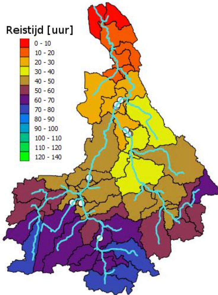
Figuur 18. Cumulatieve reistijd bij de meest voorkomende afvoer ( 1 \text{ m}^3 \text{ s}^{-1} ) van de piekconcentratie van een conservatieve opgeloste stof in de waterlopen van de Drentsche Aa naar het station De Punt in het noorden van het gebied. De reistijd voor elk substroomgebied is inclusief de reistijd binnen het substroomgebied zelf.
