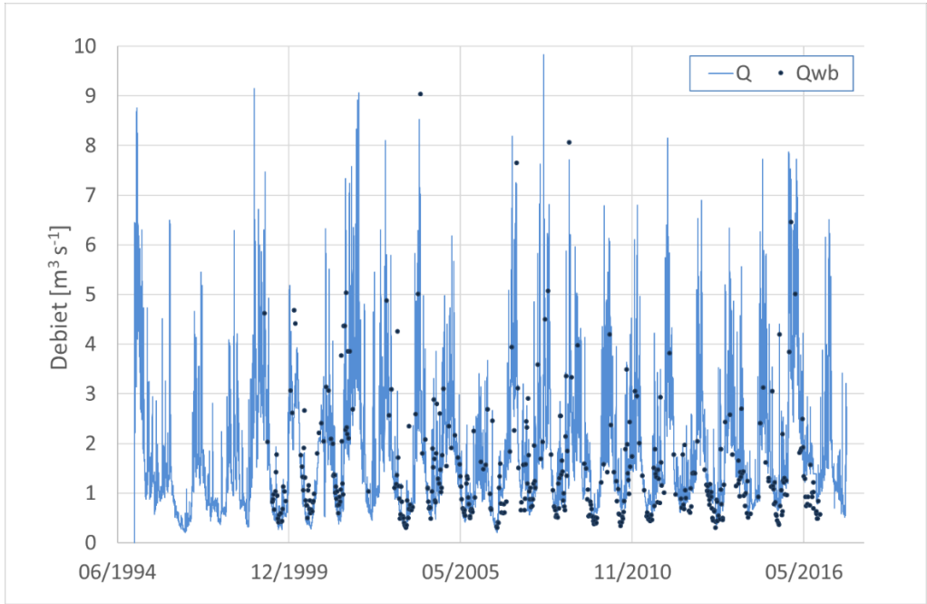
Figuur 12. Vergelijking van de nieuw berekende afvoeren (Q) met de debieten gemeten door het Waterbedrijf Groningen (Q wb ).
