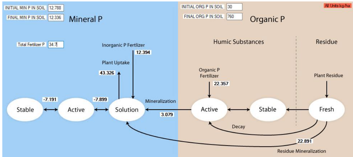
Figuur 68. Schematische weergave van de cyclus van fosfor voor het stroomgebied van de Drentsche Aa met jaarlijks gemiddelde fluxen [kg ha -1 ] voor de periode 1968-2016.
