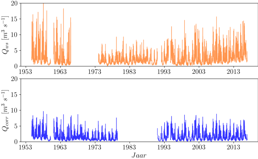
Figuur 13. Tijdseries van afvoer bij meetstation Schipborg, zoals berekend met de afvoerformule van het Waterschap Hunze en Aa's (boven), en na toepassing van de nieuw ontwikkelde QH vergelijking (onder). Het verdeelwerk Loon is in 1965 geïnstalleerd en de peilschaal is in het begin van de jaren '70 vervangen,
