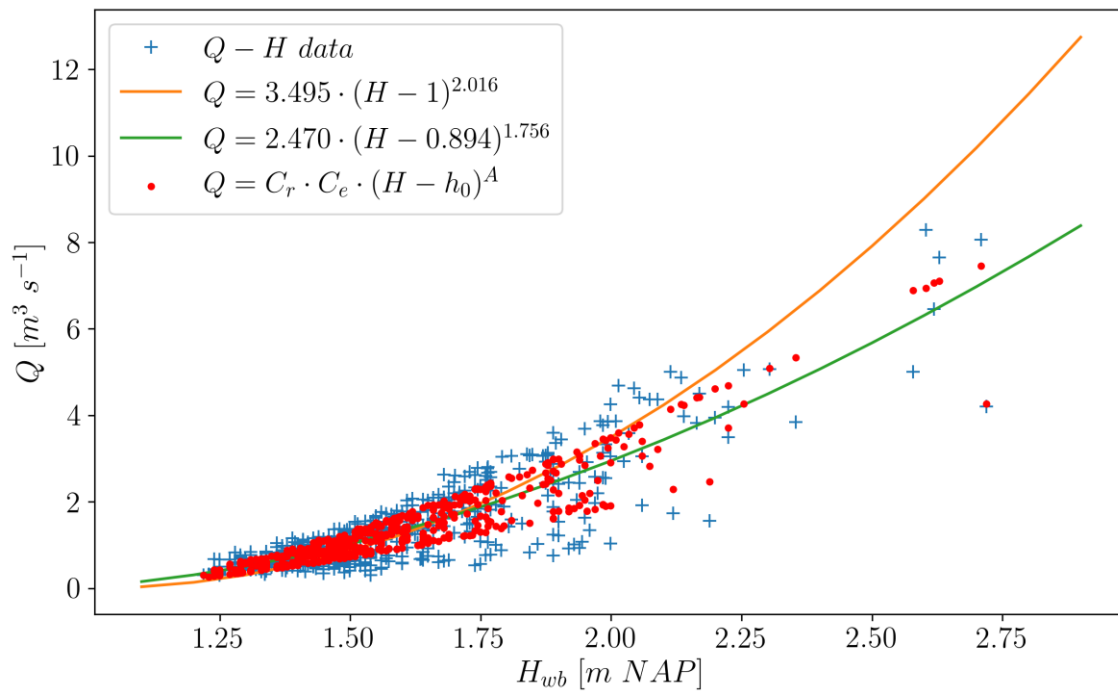
Figuur 10. Afvoer uitgezet tegen het waterpeil voor verschillende QH curves. De rode punten geven de resultaten weer indien seizoenale variatie in stroomsnelheid wordt meegenomen zoals in vergelijking 3.
