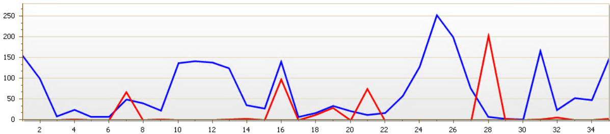
Figuur 61. Kalibratie van \text{NH}_4\text{-N} vrachten bij meetpunt De Groeve (2013-2015).
