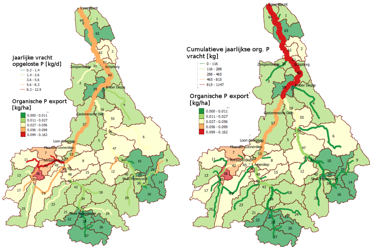
Figuur 71. Jaarlijkse export van organisch gebonden P uit substroomgebieden, vrachten van opgeloste P in waterlopen in substroomgebieden (links), en de cumulatieve vrachten van opgeloste P in de waterlopen van de Drentsche Aa (2013-2015; rechts).
