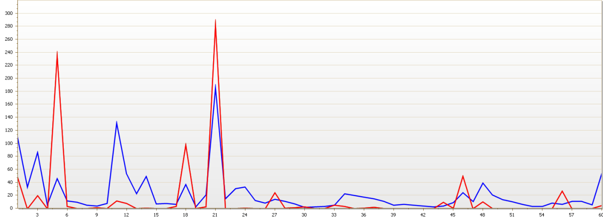
Figuur 54. Kalibratie van de vracht van P-tot [ kg d^{-1} ] bij station De Punt ( n=60 ).
