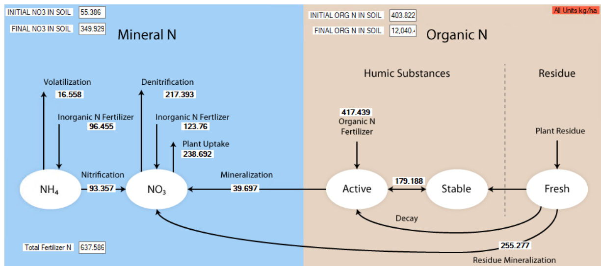
Figuur 77. Schematische weergave van de cyclus van stikstof voor het stroomgebied van de Hunze [kg ha -1 ] voor de periode 1967-2016.
