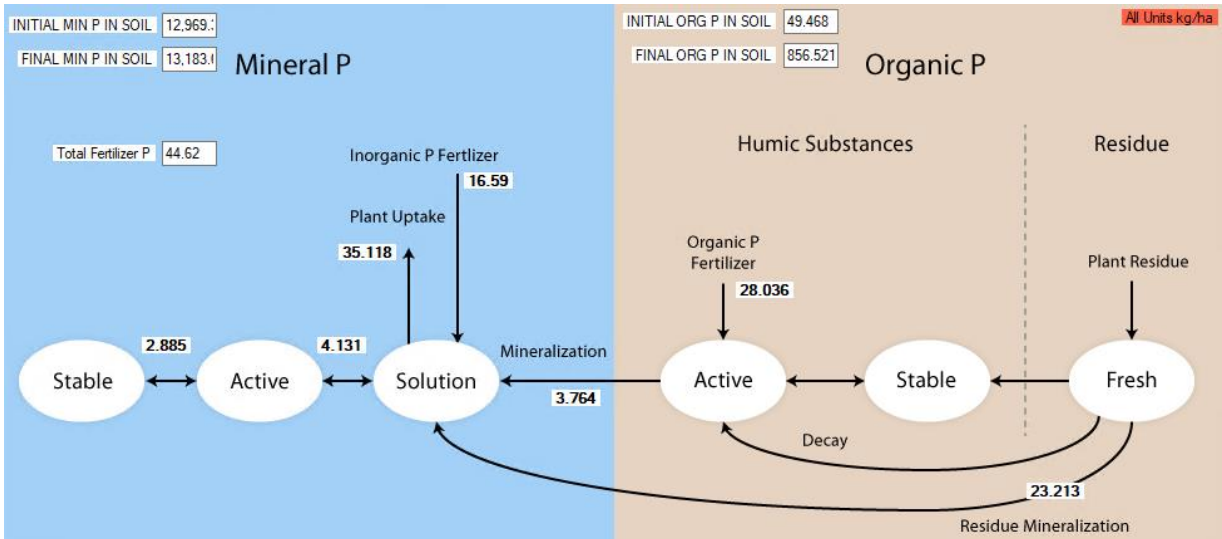
Figuur 78. Schematische weergave van de cyclus van fosfor voor het stroomgebied van de Hunze [kg ha -1 ] voor de periode 1967-2016.
