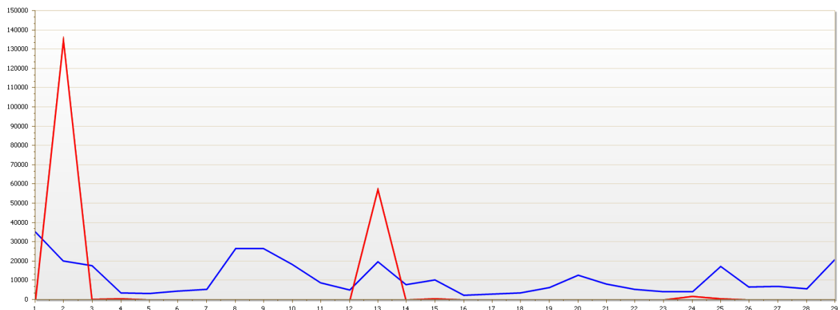
Figuur 55. Kalibratie van de vrachten van MCPA [ \text{mg d}^{-1} ] bij station De Punt ( n=29 ).
