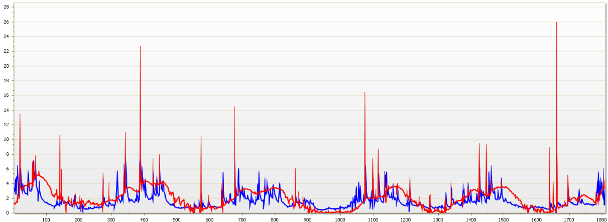
Figuur 52. Kalibratie van de afvoer [ m^3 s^{-1} ] van station Schipborg (2007-2011).
