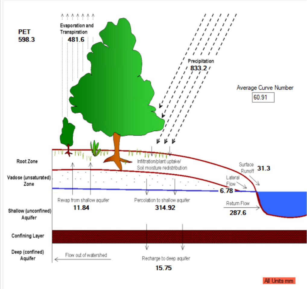
Figuur 75. Schematische weergave van de met SWAT gesimuleerde fluxen van water [ \text{mm j}^{-1} ] over de periode 1 januari 1967 tot 31 december 2016 voor het stroomgebied van de Hunze.
