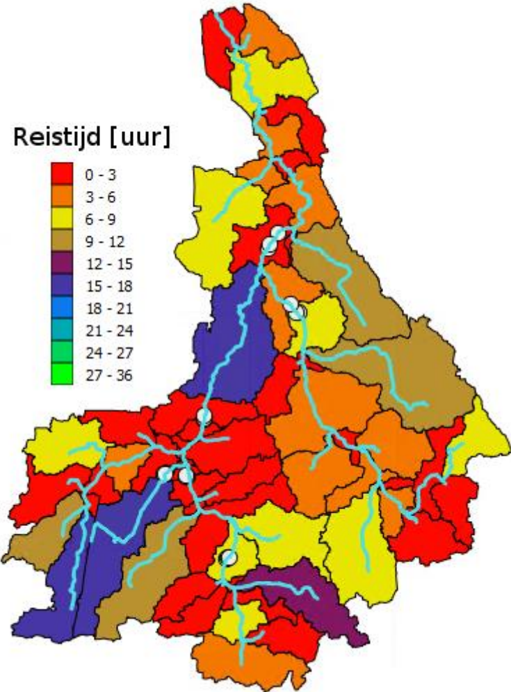
Figuur 17. Met het SWAT model gemodelleerde reistijden in de 64 substroomgebieden in het stroomgebied van de Drentsche Aa bij een afvoer bij Schipborg van 1 \text{ m}^3 \text{ s}^{-1} .
