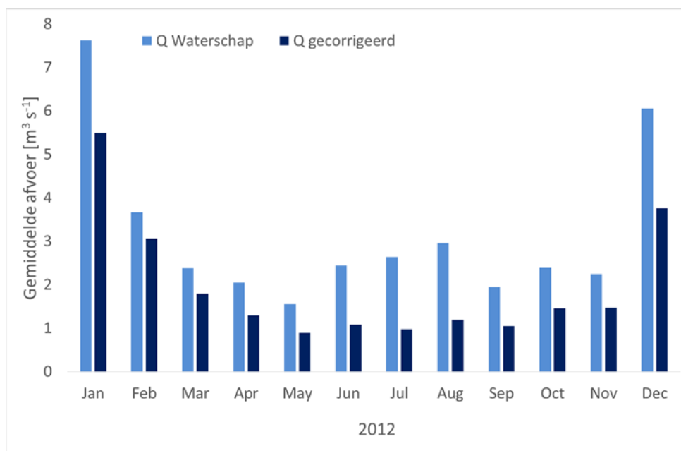
Figuur 14. Vergelijking tussen gemiddelde maandelijkse afvoer berekend met de QH vergelijking van het Waterschap, en de in deze studie ontwikkelde vergelijking.
