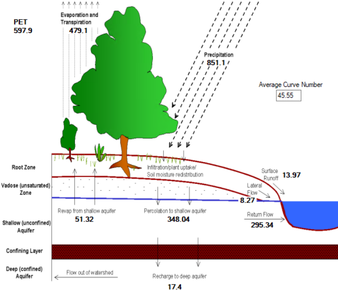
Figuur 65. Schematische weergave van de met SWAT gesimuleerde fluxen van water [mm·j -1 ] over de periode 1 januari 1967 tot 31 december 2016 voor het stroomgebied van de Drentsche Aa.
