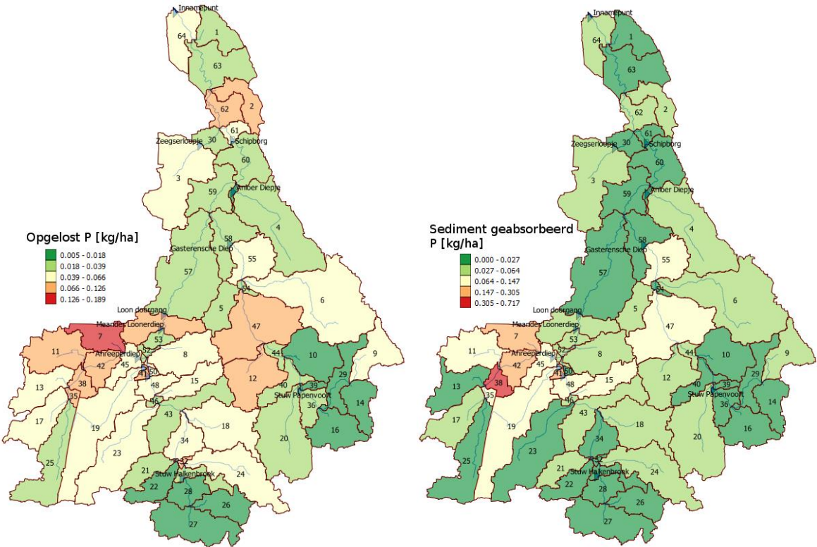
Figuur 70. Jaarlijkse export van opgelost en aan sediment gebonden P naar de waterlopen vanuit de percelen.
