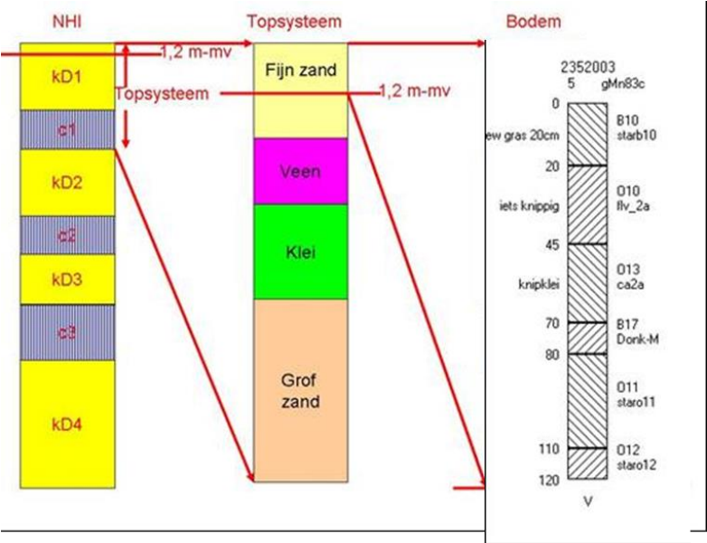
Figuur 21. In de studie 'Landsdekkende schematisering en parameterisatie van het topsysteem ten behoeve van hydrologische modellering' (Van der Gaast et al., 2015) zijn bodemprofielen verdiept door een combinatie van verschillende gegevensbronnen: voor de bovenste 1.2 tot ruim 3 m is bodemkundige informatie uit de bodemkaart en uit detailkarteringen gebruikt; tot een diepte van 5-10 m zijn deze profielen verlengt op basis van het Topsysteem (ca. 300000 boringen tot enkele meters diepte); voor grotere diepte tot 20 m is de geohydrologische opbouw uit het NHI gebruikt. Zo ontstaat een verfijning van informatie naar boven toe.
