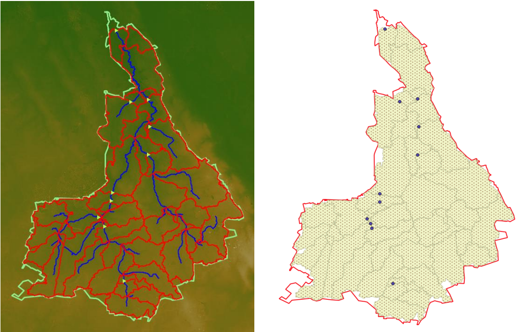
Figuur 41. Indeling van het stroomgebied van de Drentsche Aa in sub-stroomgebieden op basis van stroomgebiedsbegrenzing Waterschap Hunze en Aa's, het AHN, hoofdwatergangen en meetpunten met gebruik van de terreinanalyse routines uit MWSWAT. Het rechter figuur toont de verschillen tussen de stroomgebiedsbegrenzings van waterschap en SWAT model. De rode lijn geeft de begrenzing aan die door het Waterschap gebruikt wordt, en het gearceerde gebied geeft het stroomgebied aan zoals door terreinanalyse verkregen uit het AHN, en gebruikt in het SWAT model. De blauwe punten zijn de meetlocaties van het Waterschap.
