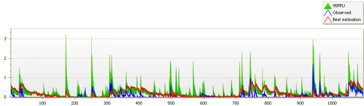
Figuur 56. Kalibratie van de afvoer van het Achterste Diep (2013-2015).
